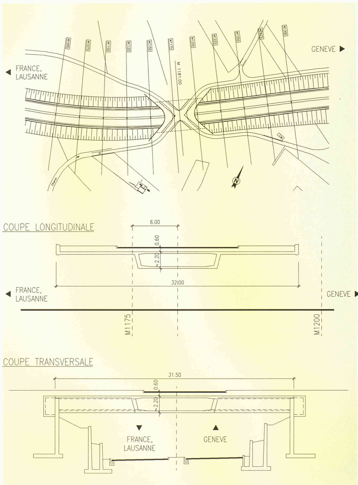
Fig. 2. – Pont des Vaulx (OA 454): étude d'avant-projet
