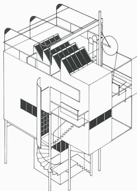
Vue axonométrique
