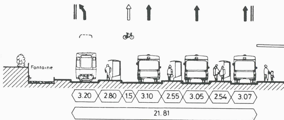
Coupe à travers la station de Cornavin
