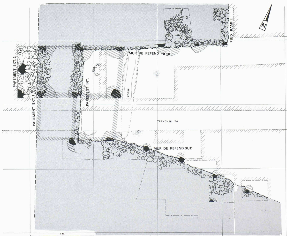
Fig. 6. – Plan archéologique de la tour sud
