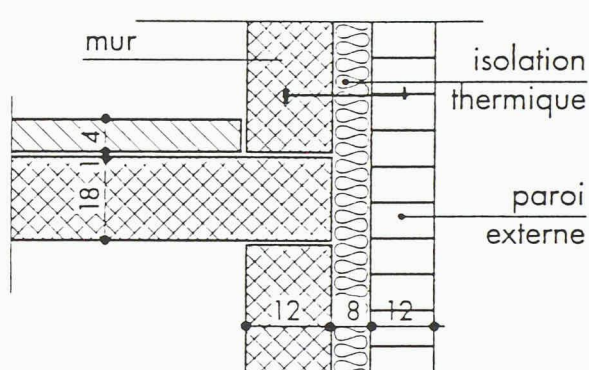
Fig. 4. - Coupe verticale d'un mur composé ou à double paroi
