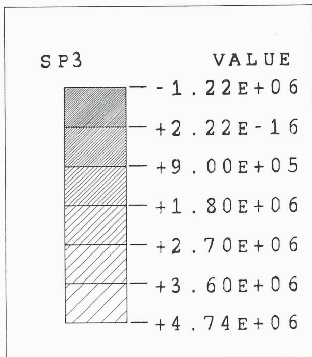
Fig. 3. – Exemple, en noir et blanc, d'échelle de couleurs rationnellement et automatiquement définie par un rapport numérique visiblement peu rationnel. La valeur de + 2.22 \text{ E}-16 est toutefois suffisamment proche du zéro pour être confondue avec celui-ci. L'indication de l'unité utilisée n'est apparemment ni requise ni nécessaire.
