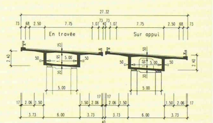
COUPE TYPE Tabliers exécutés en encoirlement (axes 13 à 18)
