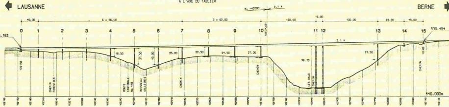
VIADUC AVAL — COUPE LONGITUDINALE
