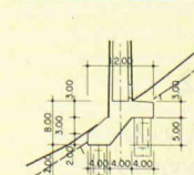
FONDATION PILE 13
