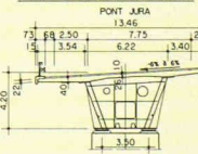
COUPE TRANSVERSALE
