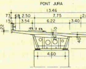
COUPE TRANSVERSALE
