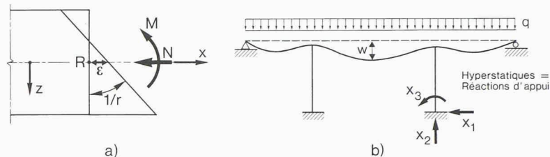
Fig. 3. – Définition de la courbure, de la déformation relative et de la déformée d'une structure linéaire: a) déformation relative et courbure d'une section; b) calcul de la déformée par intégration des courbures des sections
