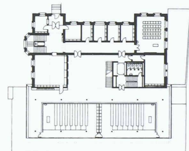
Rez-de-chaussée
