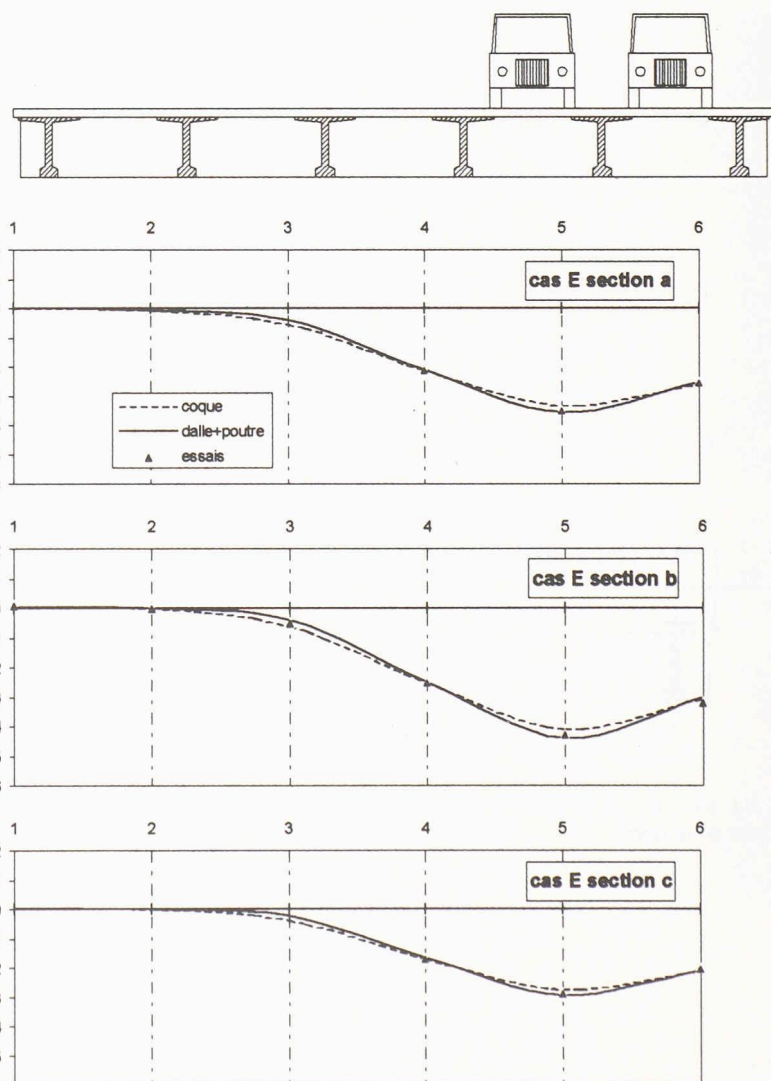
Fig. 19. Déformées transversales de la travée 5 pour le cas de charge E
