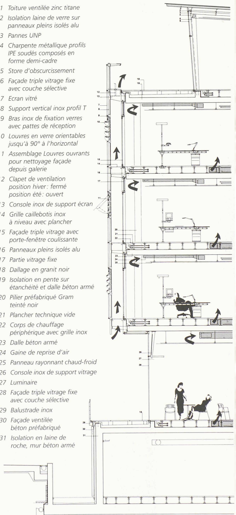
Coupe technique, façade est
