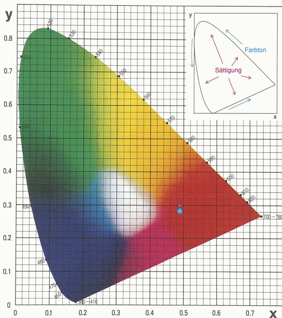
Triangle de la norme de la Commission Internationale de l'Éclairage (CIE 1931): Sättigung = saturation, Farbton = nuance Photo Minolta S.A., Dietikon
