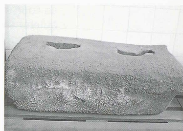
Fig. 2. – Anode endommagée par une combustion au \text{CO}_2
