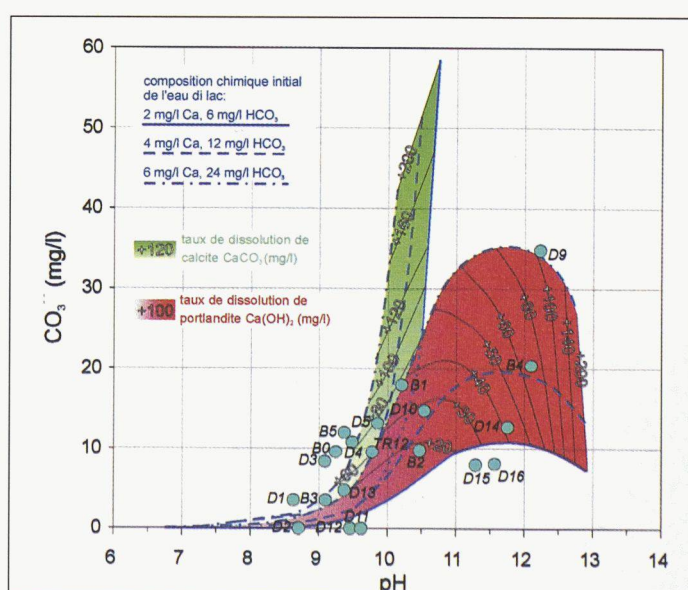
Fig. 5. - Diagramme \text{pH}-\text{CO}_3^{2-} avec les domaines de dissolution de portlandite (en rouge) et de calcite (en vert) par rapport au chimisme de l'eau du lac, avec \text{pH} et concentration en \text{CO}_3^{2-} des eaux sortant des drains. Les drains dans le domaine de la portlandite témoignent d'une dissolution de l'écran d'étanchéité
