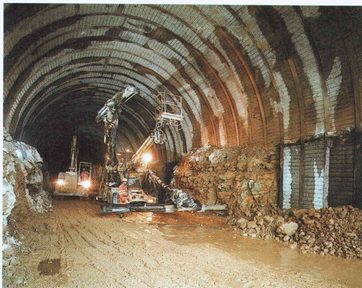
Tunnel de La Raisse (1250 m) (Photo C. Cuendet)
