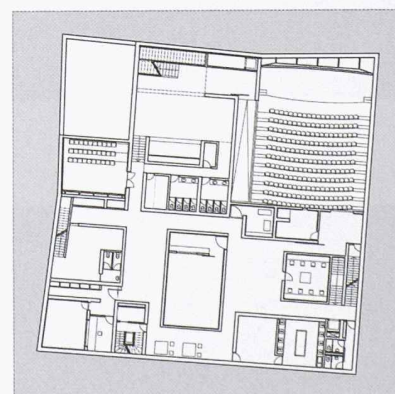
PLAN DU SOUS-SOL (niveau -540)
