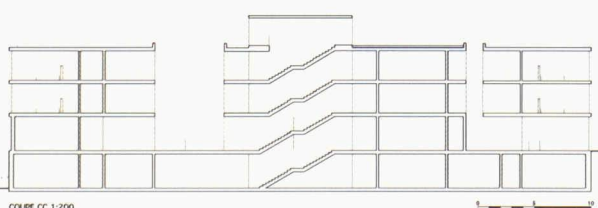
COUPE CC 1:200
