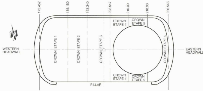
Exécution des plans d'armature de la caverne principale
