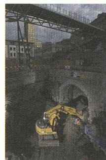
Attaque du tunnel St-Laurent (Photo métro m2 / Maurice Schobinger)
