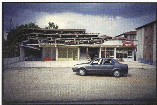
Izmit, après le séisme du 17 août 1999 (Photo SGEB, Société Suisse du Génie Parasismique et de la Dynamique des Structures)
