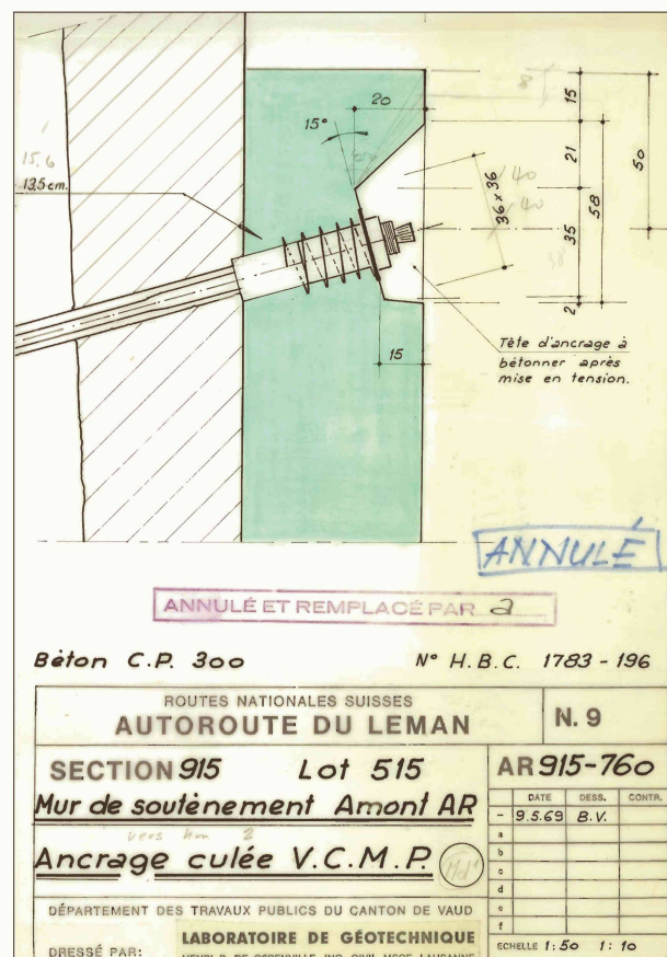
Fig. 2 : Exemple de document d'archive illustrant la difficulté à se faire une idée de ce qui a réellement été mis en œuvre en matière d'ouvrage ancré
