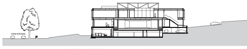
COUPE TRANSVERSALE B
