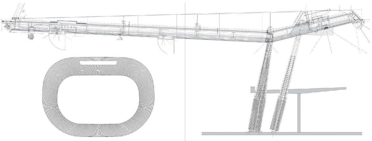
Détail constructif de la toiture, Stade du Letzigrund (Béatrix & Consolascio)
