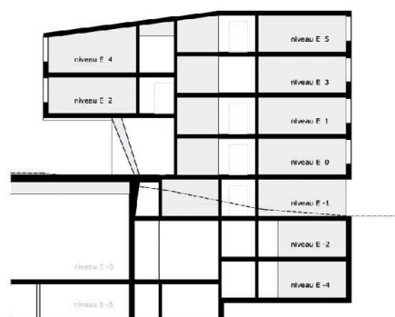
Bât.E : coupe sur l'entrée
