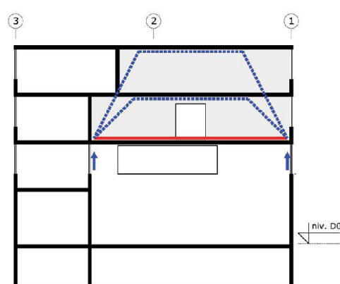
Bât.D : coupe axe C-C
