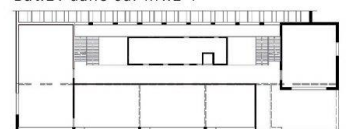
Bât.E : dalle sur niv.E-1
