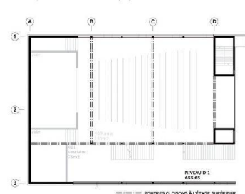
Bât.D : niv.1 « Aula »
