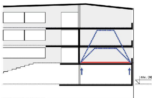
Bât.D : coupe axe 2-2
