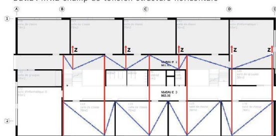
Bât.E : niv.2 champ de tension structure horizontale
