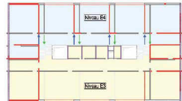
Bât.E : réactions horizontales des dalles
