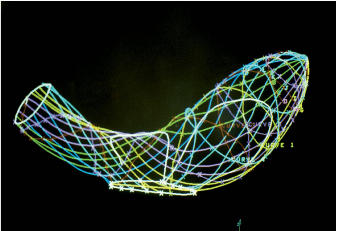
Frank O. Gehry & Associates, Inc. Résidence Lewis, Lyndhurst, Ohio : Poisson, maquette 3D Catia de la géométrie de la véranda, 1989-1995 (Image fournie par Gehry Partners, LLP)
