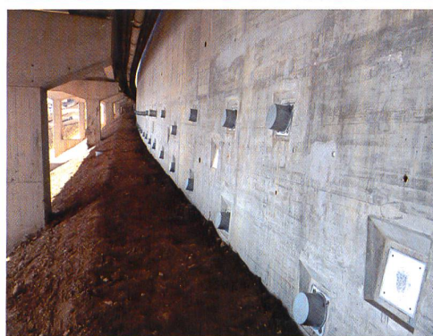
A9 – Les Curnilles: renforcement d'un mur aval à semelle (photo GUMA)
