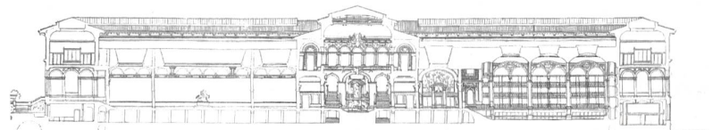
Fig. 8. — Coupe longitudinale. — Echelle : 1 : 600.
