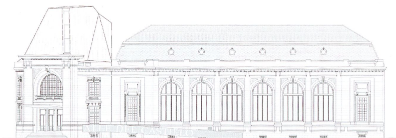
Façade Nord
