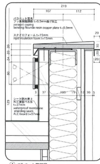
① パラペット詳細図 parapet detail S:1/5
