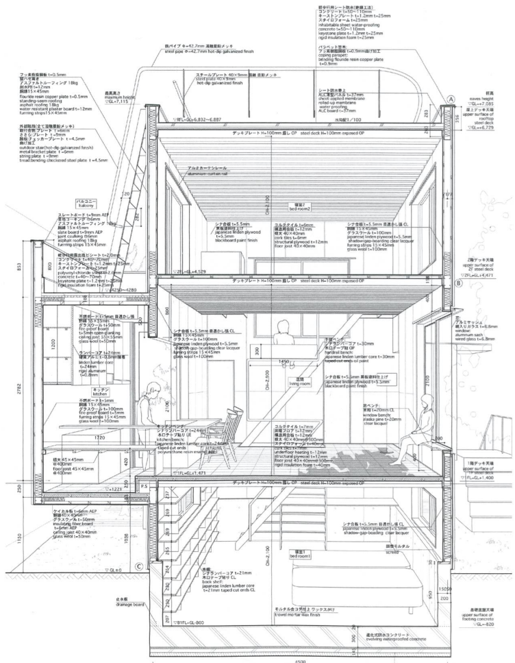
断面詳細パース vertical section perspective S:1/30
