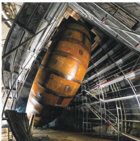
Coude de la conduite blindée au bas de l'un des deux puits verticaux de la centrale de pompage-turbinage de Nant de Drance (photo Nant de Drance SA)
