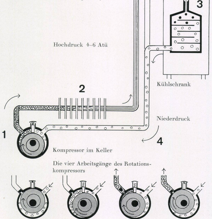
Die Arbeitsgänge im Kompressor-Kühlschrank (Rotationskompressor)
