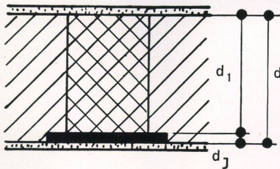
Abb. 2 Beiderseits verputzte, ohne Putz 32 cm dicke Mauer aus Hohlsteinen ( \lambda = 0,41 ), mit nach innen zu durch eine Korkschiebt ( \lambda_2 = 0,04 ) abisolierter Eisenbetonsäule ( \lambda_1 = 1,3 ).
