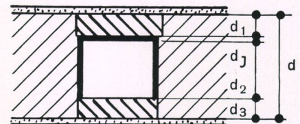
Abb. 4 Beiderseits verputzte, ohne Putz 32 cm dicke Mauer aus Hohlsteinen ( \lambda = 0,41 ), mit einem etwa 17 cm tiefen Luftschlitz, der nach außen durch eine Korkschiebt ( \lambda_2 = 0,04 ) und 6 cm dicke Isoliersteine ( \lambda_1 = 0,51 ), nach innen durch eine 6 cm dicke Isolierplatte ( \lambda_3 = 0,25 ) abgedeckt ist.
