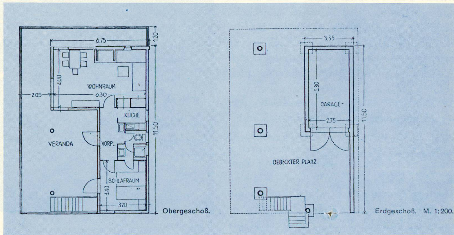
Grundriß Wohngeschoß und Untergeschoß
