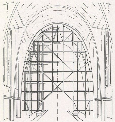
Fahrbares Schalungsgerüst für die projektierte katholische Maria-Friedenskirche in Dübendorf. Architekten Pfammatter & Rieger, Zürich.
