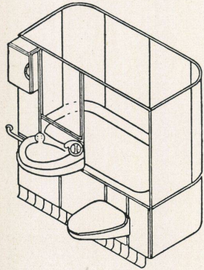
10 Französischer Installationsblock; Wanne, Klosett, Waschtisch und Toiletenschrank sind mit den Umfassungswänden zu einem transportablen Stück in der Fabrik zusammengestellt. Auf der Baustelle sind nur noch obere und untere Rohranschlüsse zu erstellen.
