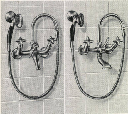
5a Neue Badebatterien mit rundem und fächerförmigem Auslauf, sowie schrägstehenden Oberteilen. Fabrikant: Aktiengesellschaft Oederlin & Cie., Armaturfabrik, Baden
