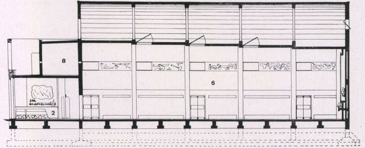
Längsschnitt / Coupe longitudinale / Longitudinal section
