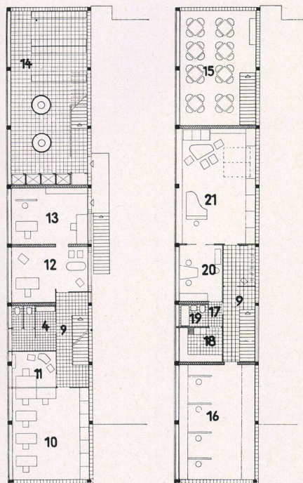
Grundrisse Bürotrakt, links 1. Obergeschoß, rechts 2. Obergeschoß / Plans du bâtiment des bureaux, à gauche 1er étage, à droite 2e étage / Plans of the office building, left, 1st upper floor, right, 2nd upper floor 1:350
