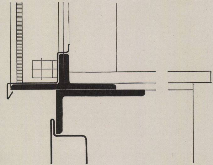
Detail A-A
