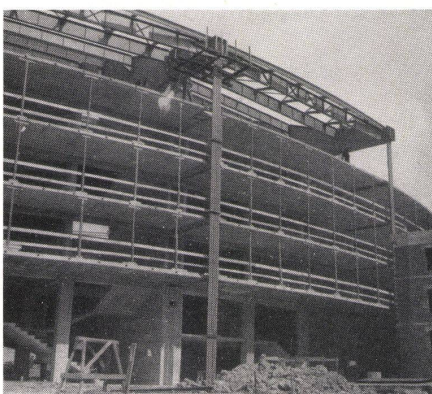
Stahlzuganker der Stahlbinder an der Außenfront. Tirant en acier des fermes à l'extérieur du stade. Steel tie rod of the steel trusses at the outside of the front wall.
