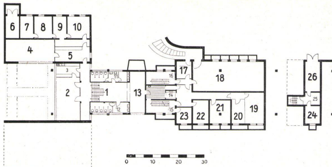
Grundriß Kellergeschoß / Plan du sous-sol / Basement plan
