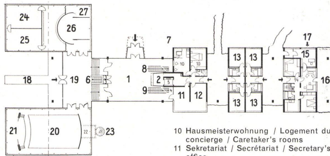
Grundriß Erdgeschoß / Plan du rez-de-chaussée / Ground-floor plan
