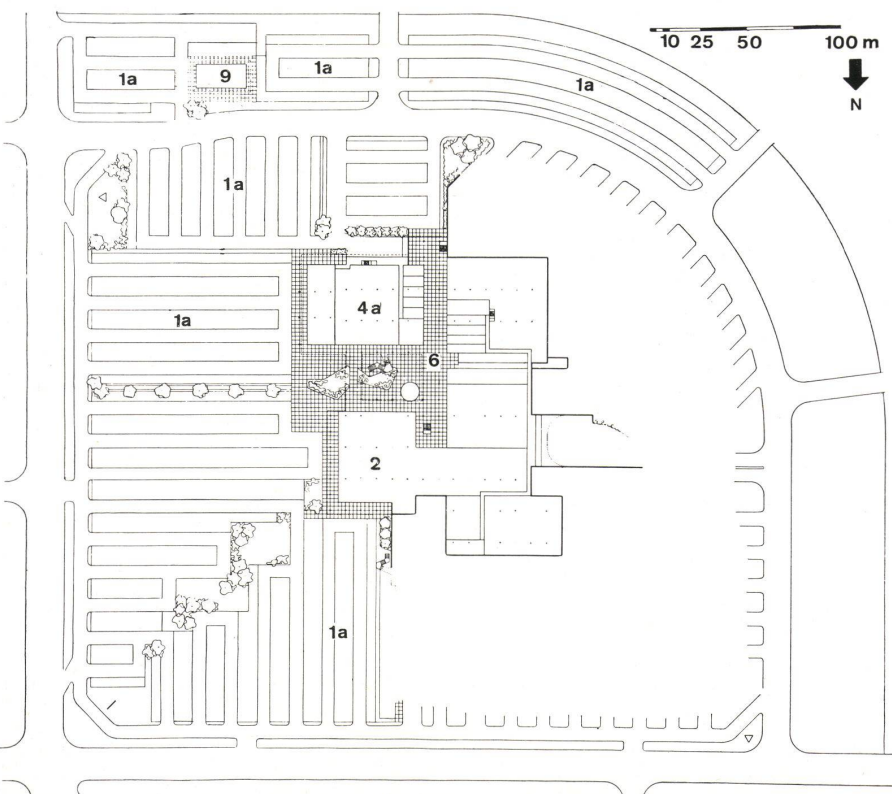
Unteres Geschoß / Etage inférieure / Lower level plan
