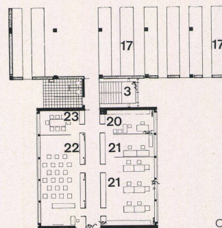
C Grundriß Obergeschoß Verwaltungsgebäude / Plan de l'étage supérieur du bâtiment administratif / Upper-floor plan of administration building 1:500
