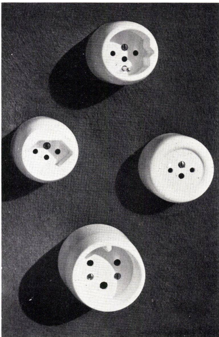
Abb. 7 (von oben nach unten) Steckdosen der neuen X-Serie 221140 ws 10 A 250 V 226130 ws 10 A 250 V 221130 ws 10 A 250 V 261130 ws 15 A 500 V Xamax AG., Zürich-Oerlikon
