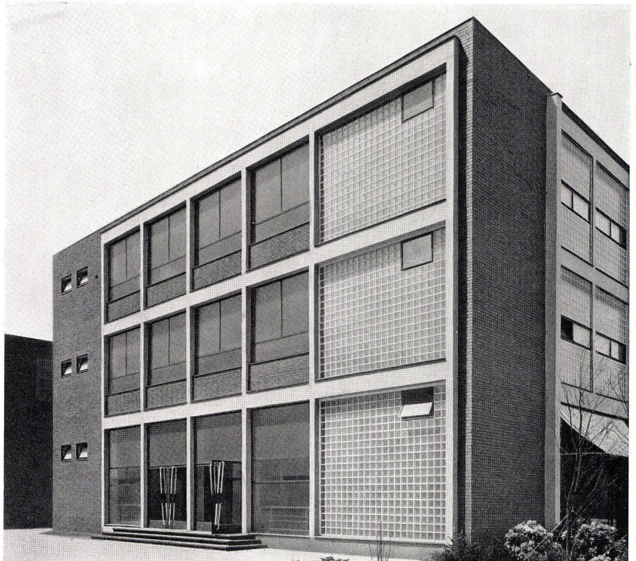
2 Ostfassade mit einem der Eingänge. Hinter den Glasbausteinen liegt das Treppenhaus. Façade est avec l'une des entrées. La cage d'escalier est située derrière les briques en verre. East elevation with one of the entrances. The stair-well is situated behind the glass bricks.
