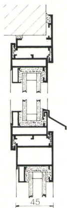
Abb. 8 Vertikalschnitt durch Drehflügelpartie vom Bürofenster, System «Menziken» (Pat. ang.), Größe Ia, für Einfach- oder Isolierverglasung, mit oder ohne Gummidichtung. (Eine Profilserie Größe II mit 56 mm Höhe steht ebenfalls zur Verfügung.) Fabrikation durch die Metallbauunternehmen und Schlossereien.
