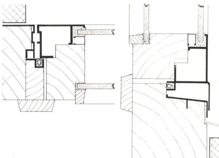
Abb. 18 Links: Horizontalschnitt, rechts: Vertikalschnitt durch Schwingflügel «Aluh», System «Schmidlin». Kombination Holz/Leichtmetall. Äußerer Flügel in Leichtmetall.
