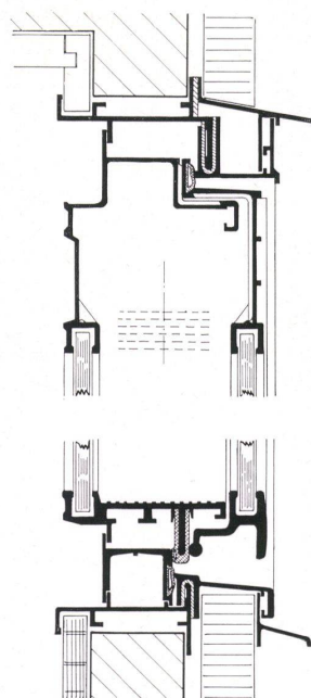
Abb. 21 Vertikalschnitt durch «Elumin»-Schwingflügel, Erstes in der Schweiz hergestelltes Ganz-Leichtmetall-Isolierfenster. Flügel und Rahmen zweiteilig mit Isolationszwischenlage und Dichtungsprofilen (In- und Ausland-Patente). Fabrikation: Gauger & Co. AG., Zürich; Hans Kießling, Eisenbau AG., Bern; Vohland & Bär AG., Riehen/Basel; Hartmann & Co. AG., Biel; Kronenberger Söhne, Luzern.
