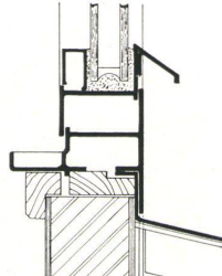
Abb. 10 Vertikalschnitt durch Drehflügelpartie vom Bürofenster, System «Hirsch», für Einfach- oder Isolierverglasung. Fabrikation: Metallbau Hirsch, Biel.
