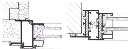
Abb. 22 Horizontalschnitt durch Drehflügel vom Isolierfenster «Alku», pat. System «Hirsch». Außen tragende Profile in Leichtmetall, innen Abdeckung mit Kunststoffprofilen. Mit oder ohne Dichtungsprofilen. Fabrikation: Metallbau Hirsch, Biel.
