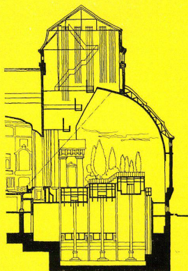
Schnitt durch die Bühne des Schauspielhauses Dresden (1910). Die Bühne hat einen festen Rundhorizont und komplizierte Versenkeleinrichtungen, die die Dekorationen ins Untergeschoß verschieben können, da Seitenbühnen auf Bühnenhöhe fehlen.
