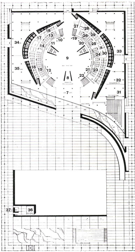
Erdgeschoß 1:3200 Rez-de-chaussée. Ground-floor.
