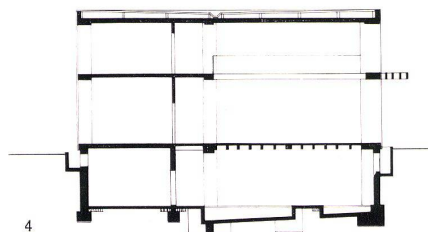
4 Querschnitt Versuchslaboratorium »Stein« 1 : 350. Coupe transversale du laboratoire d'essai «Pierre». Transverse section of the "stone" research laboratory.
