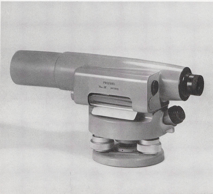
4 Nivellierinstrument. Hersteller Etablissement Fogeli SA, Brüssel. Niveau à lunette. Levelling instrument.
