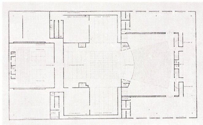
Entwurf Weber. Grundriß Foyergeschoß.
